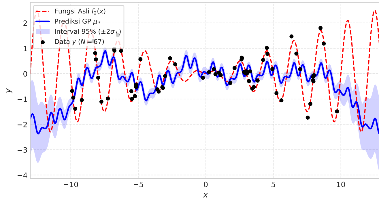
(c) Penjumlahan: k_{\text{Lin}} + k_{\text{Per}}
