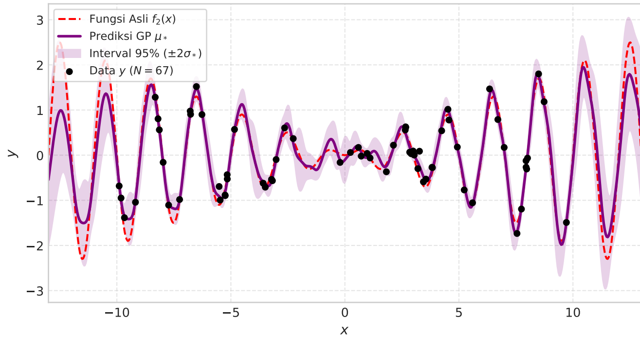
(d) Perkalian: k_{\text{Lin}} \times k_{\text{Per}}
